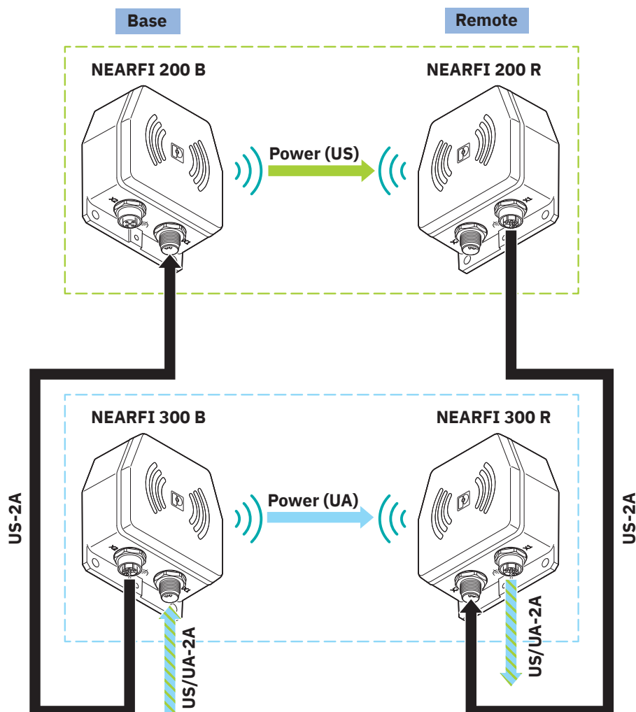
Disegno schema
