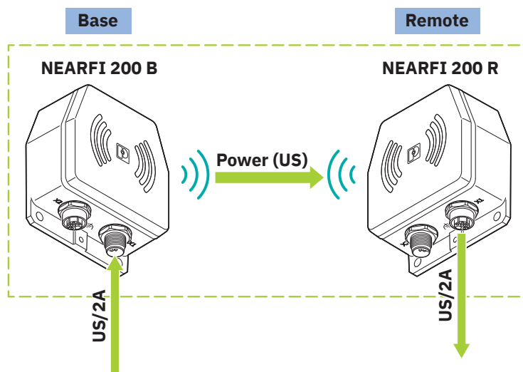
Disegno schema
