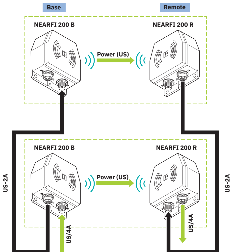
Disegno schema
