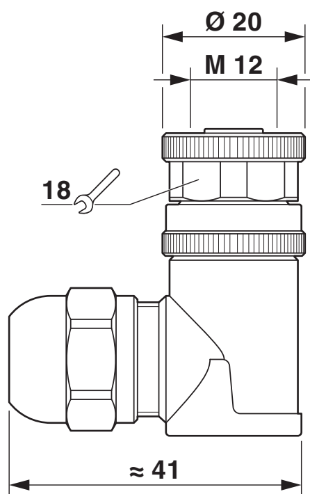
Disegno quotato
