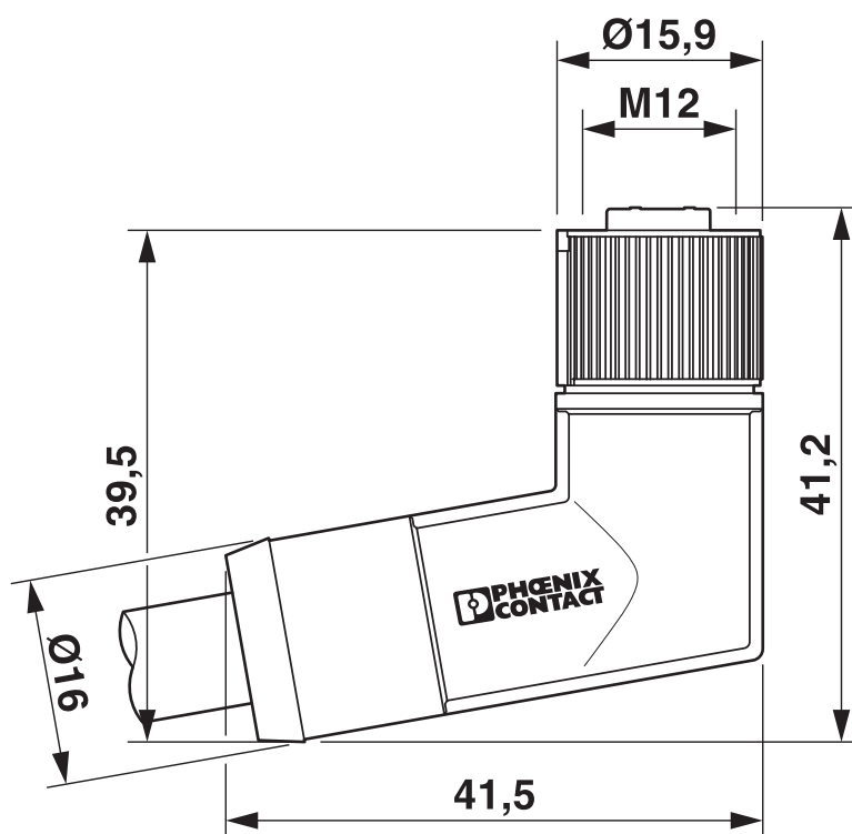
Disegno quotato
