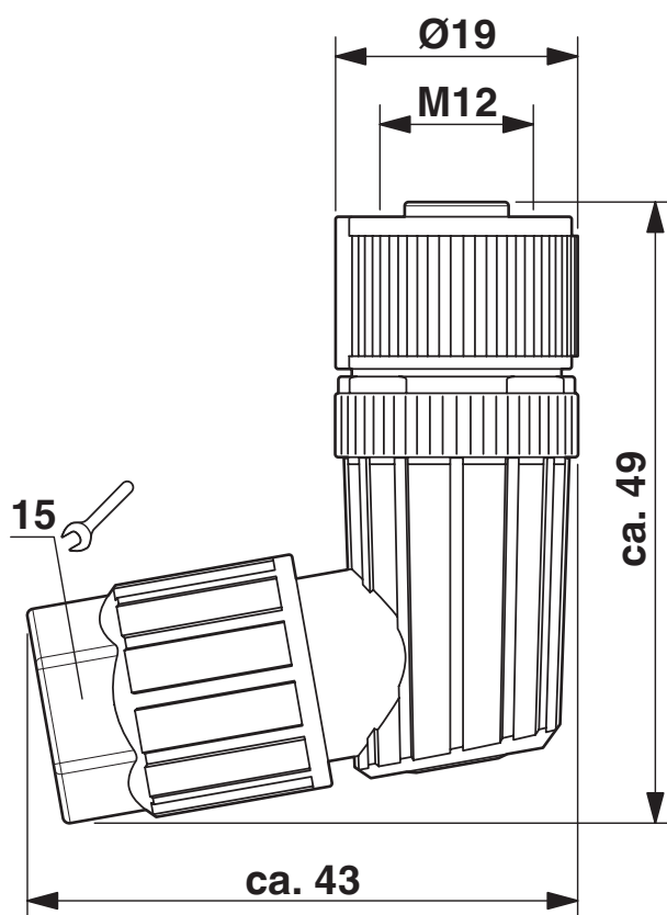
Disegno quotato
