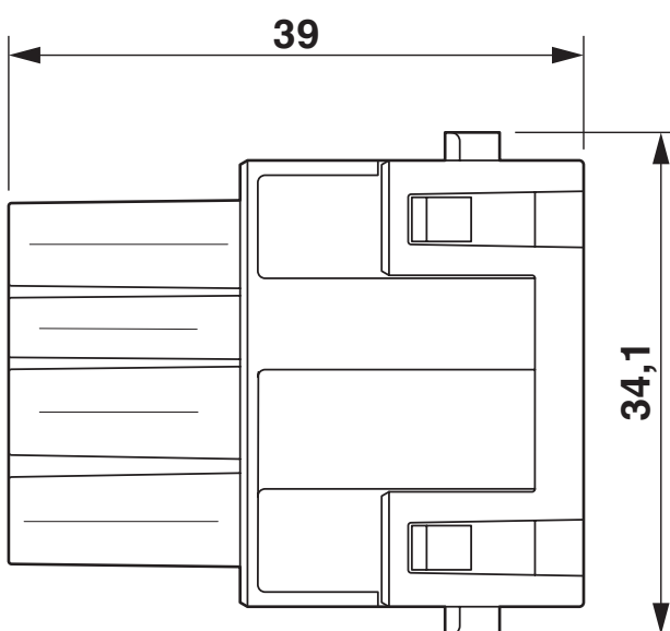
Disegno quotato
