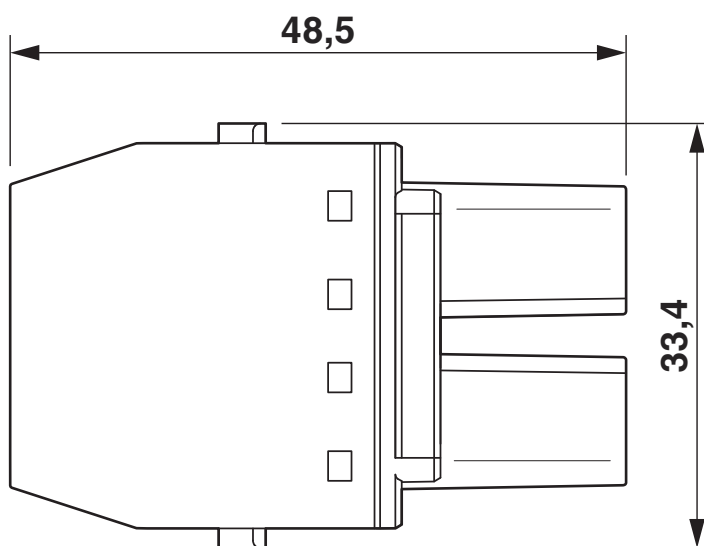
Disegno quotato
