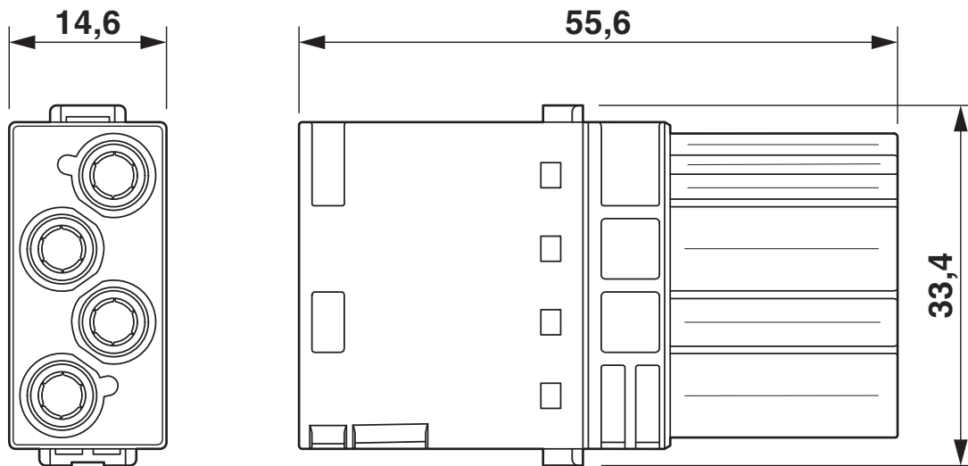
Disegno quotato
