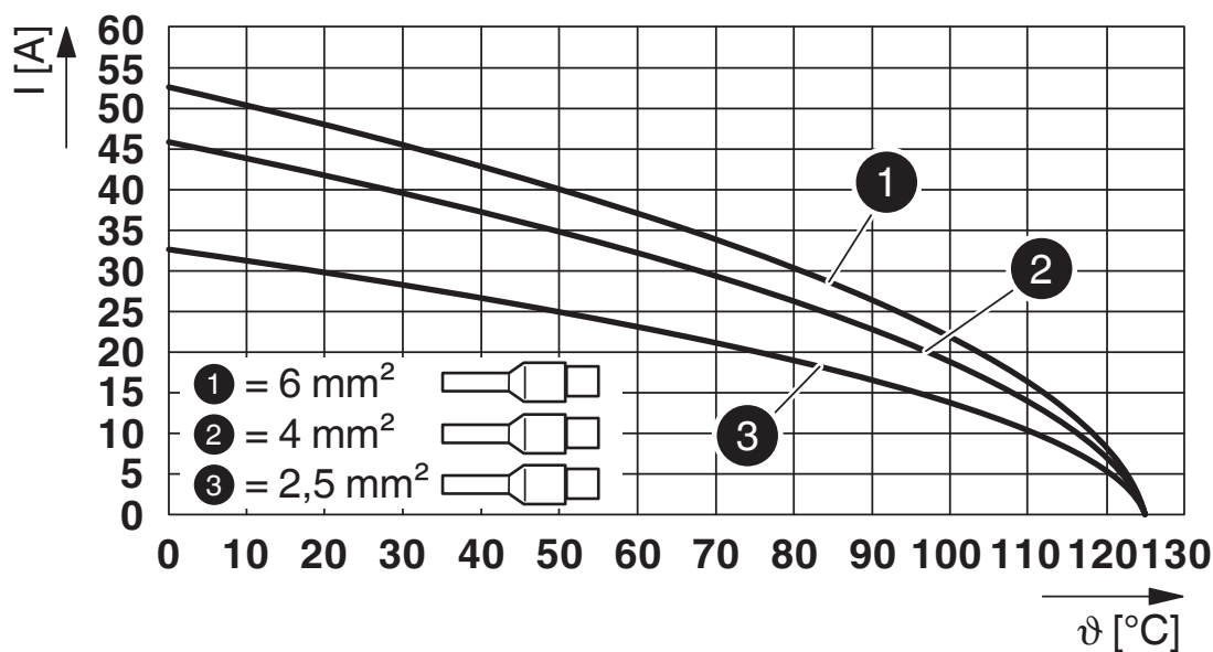
Diagramma di derating per conduttori flessibili con capocorda
