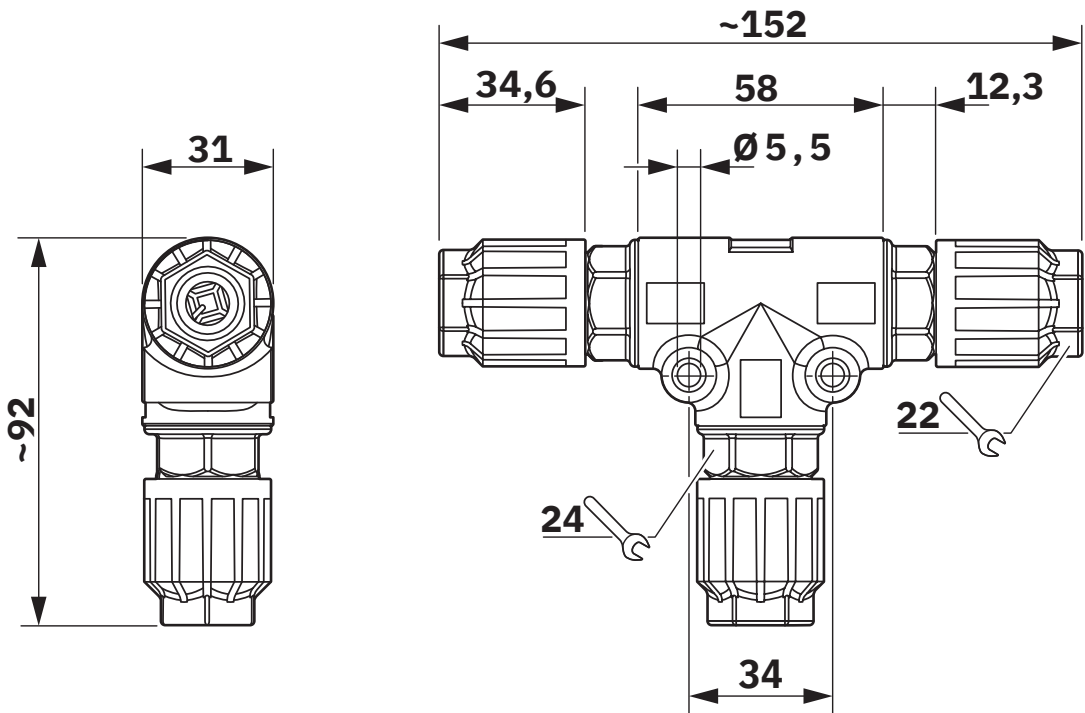
Disegno quotato
