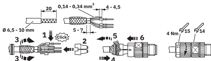
Disegno funzionamento
