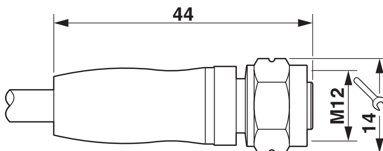
Disegno quotato
