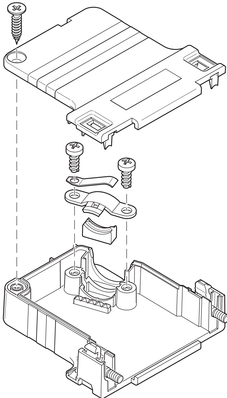
Disegno schema
