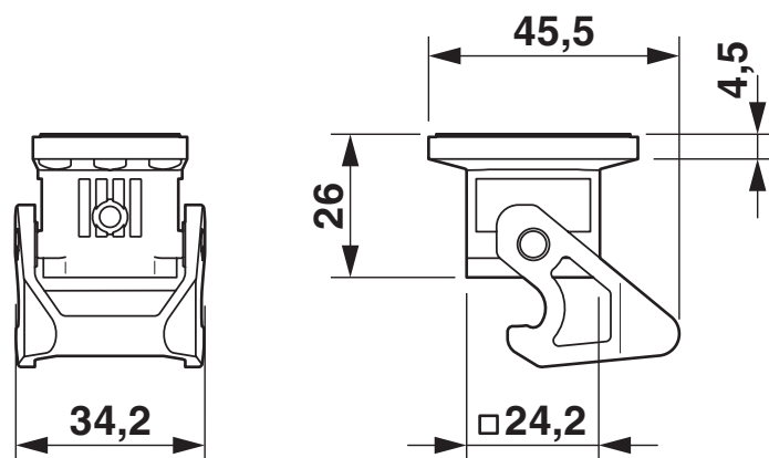
Disegno quotato
