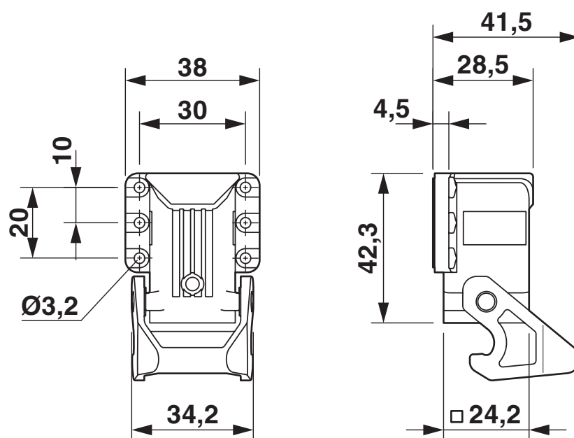
Disegno quotato
