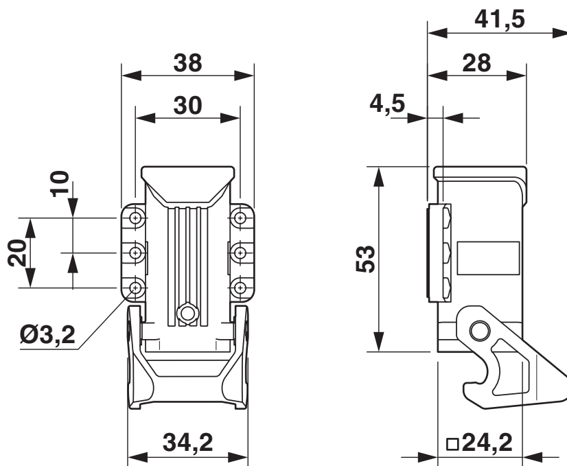
Disegno quotato
