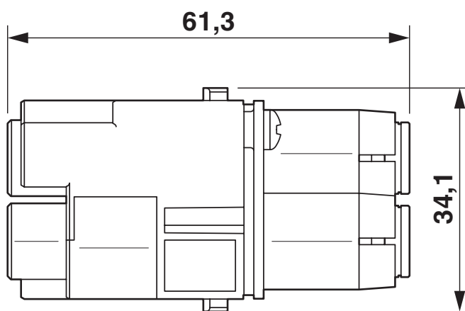
Disegno quotato
