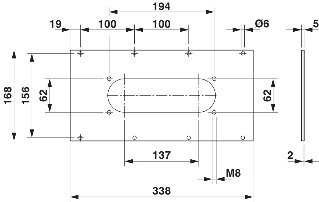
Disegno quotato
