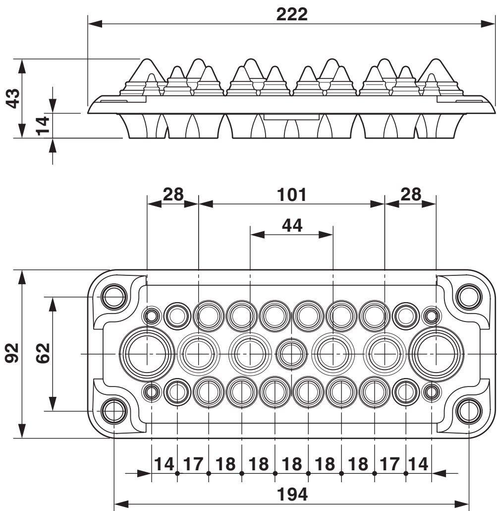
Disegno quotato
