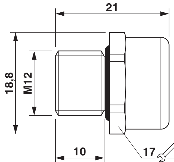
Disegno quotato
