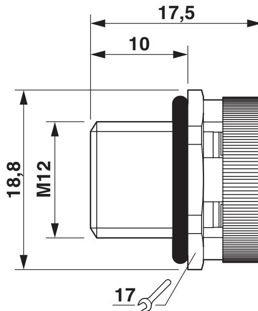
Disegno quotato
