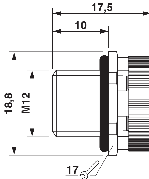
Disegno quotato
