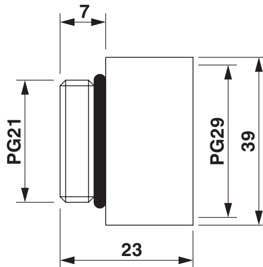
Disegno quotato
