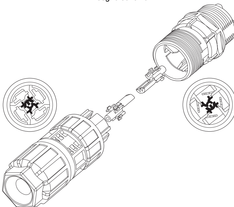
Disegno schema
