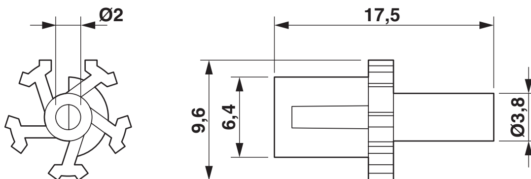
Disegno quotato
