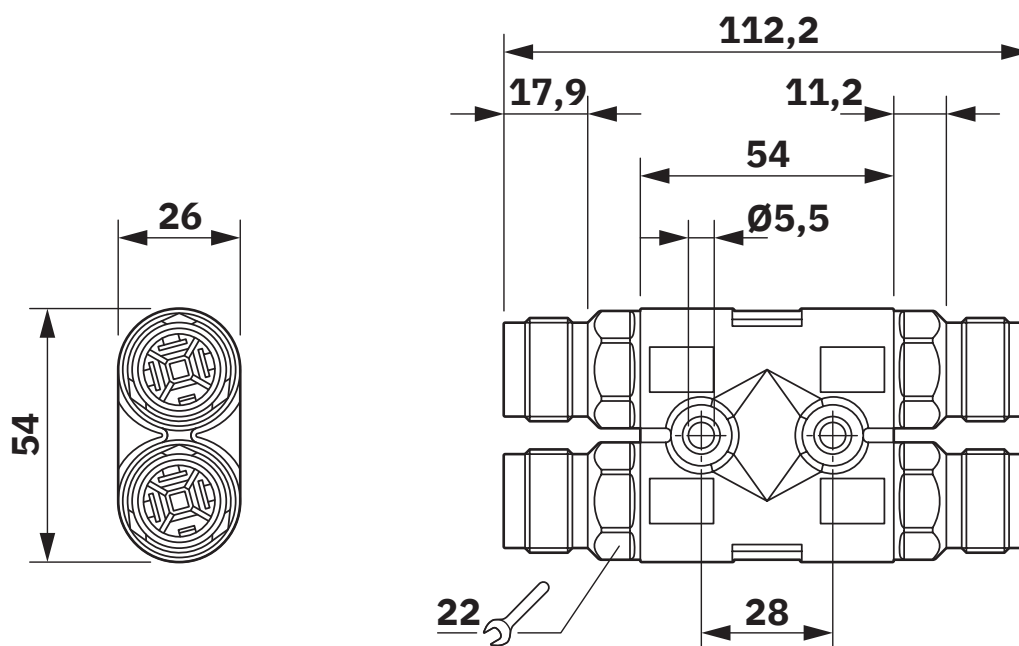
Disegno quotato
