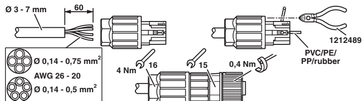
Disegno funzionamento
