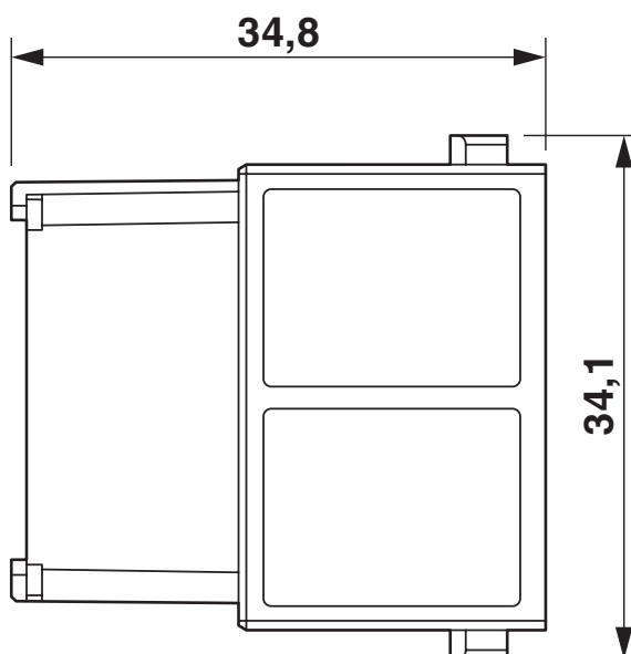
Disegno quotato
