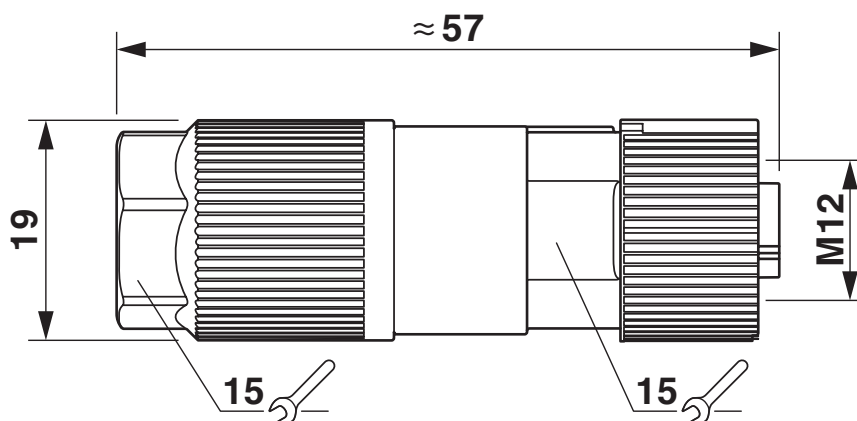
Disegno quotato
