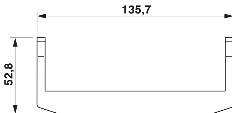
Disegno quotato
