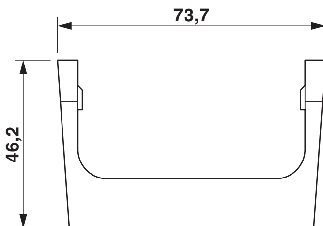
Disegno quotato
