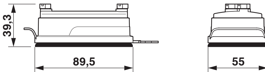
Disegno quotato
