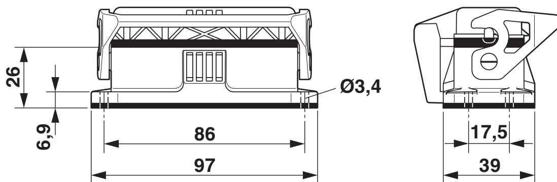
Disegno quotato
