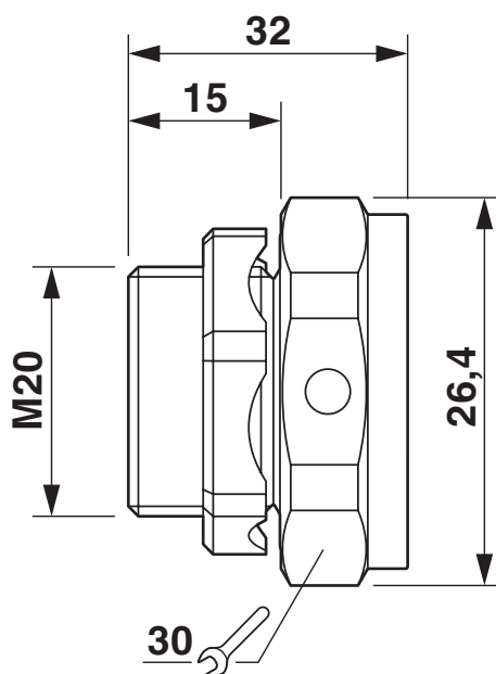
Disegno quotato
