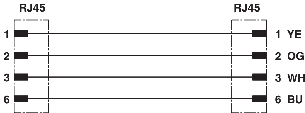
Pinning contatti del connettore RJ45
