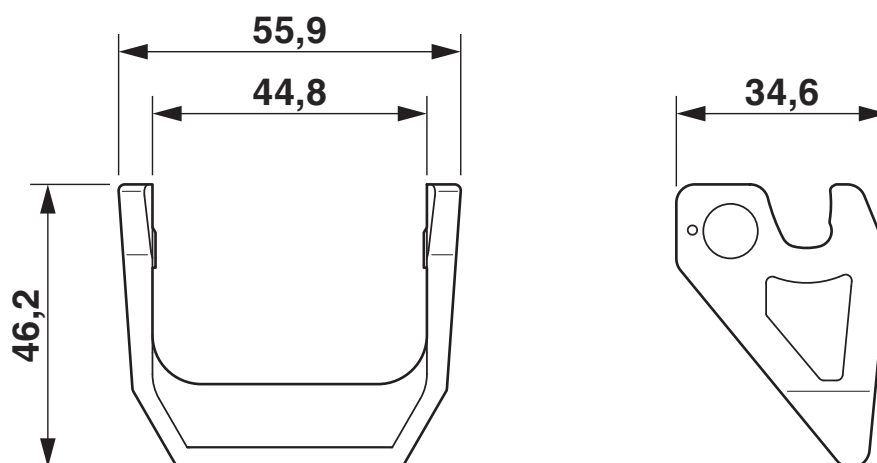
Disegno quotato
