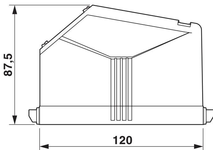
Disegno quotato
