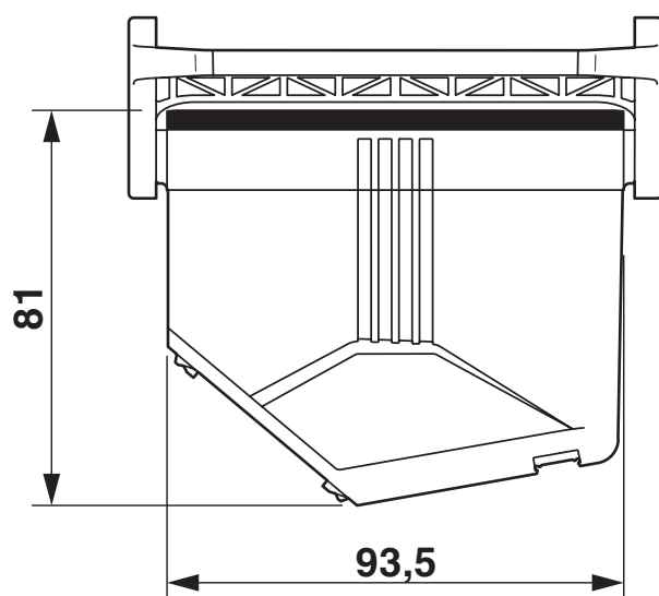
Disegno quotato
