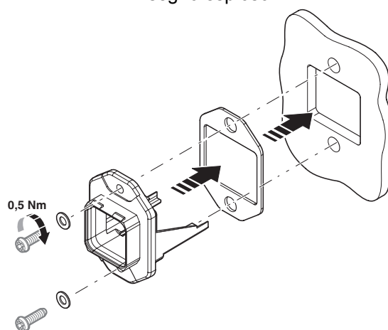
Disegno esploso
