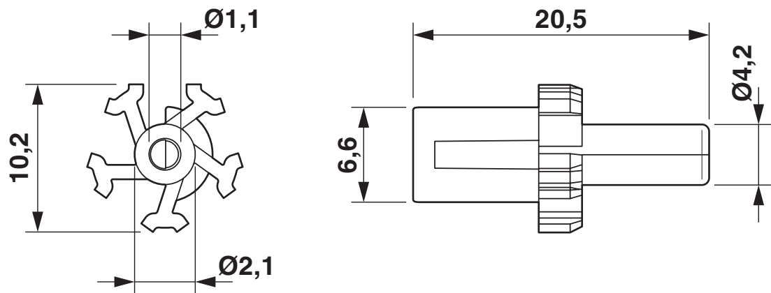
Disegno quotato
