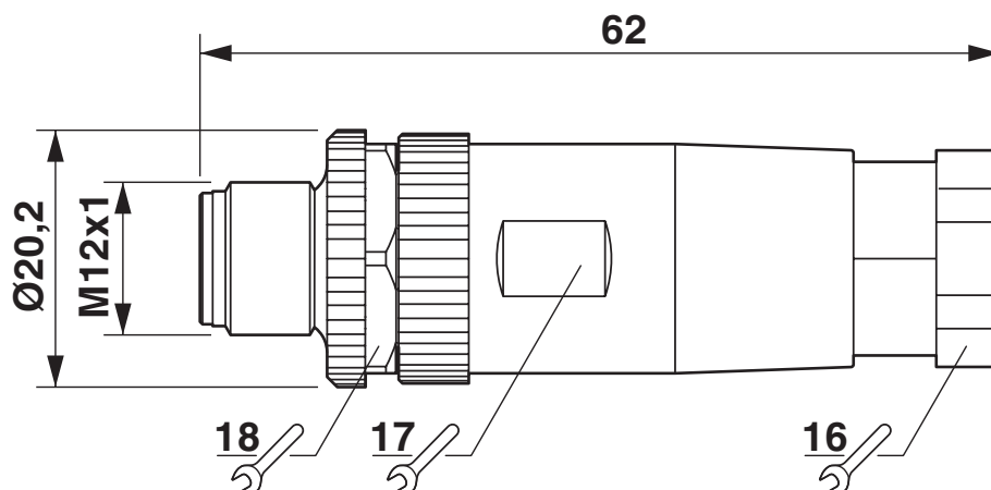
Connettore M12 x 1, diritto, schermato
