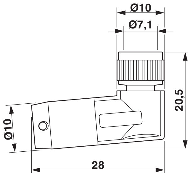
Disegno quotato
