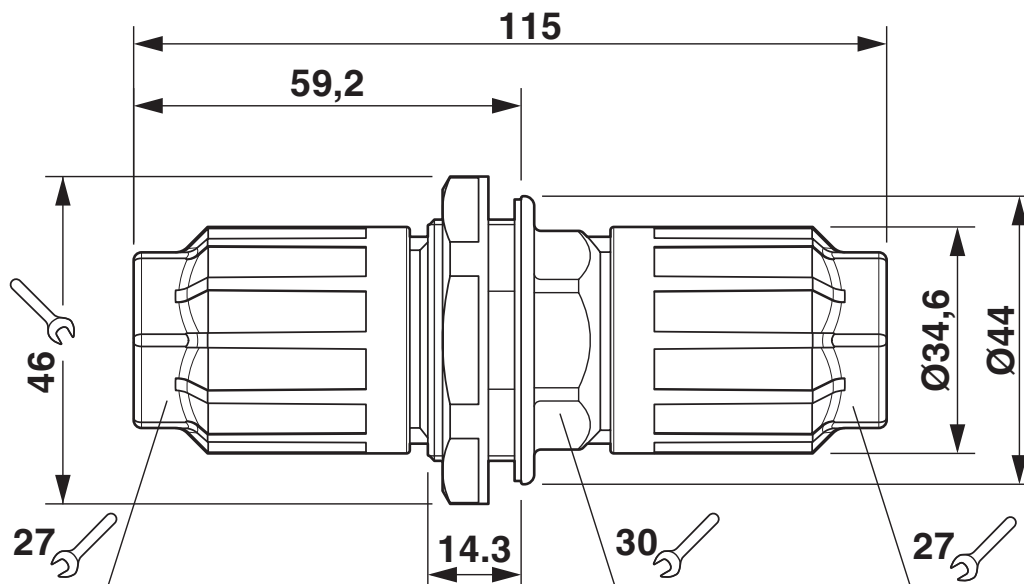
Disegno quotato
