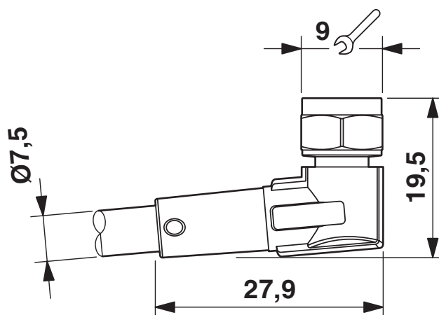
Disegno quotato
