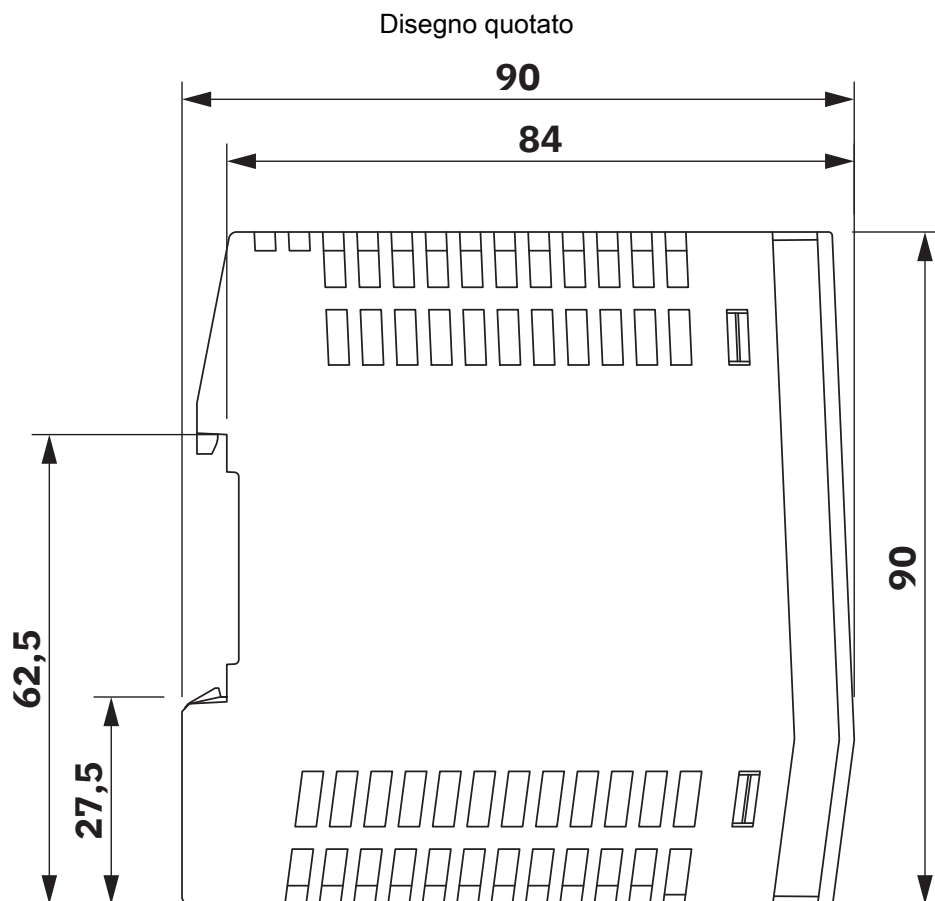
Dimensioni del dispositivo (misure in mm)
