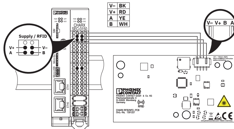
Disegno applicazione
