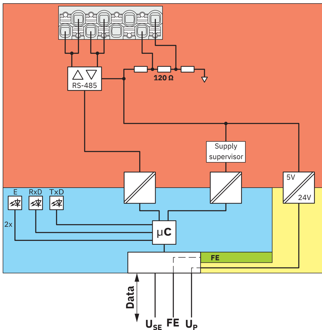
Circuito interno dei punti di connessione
