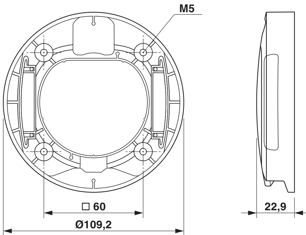
Disegno quotato
