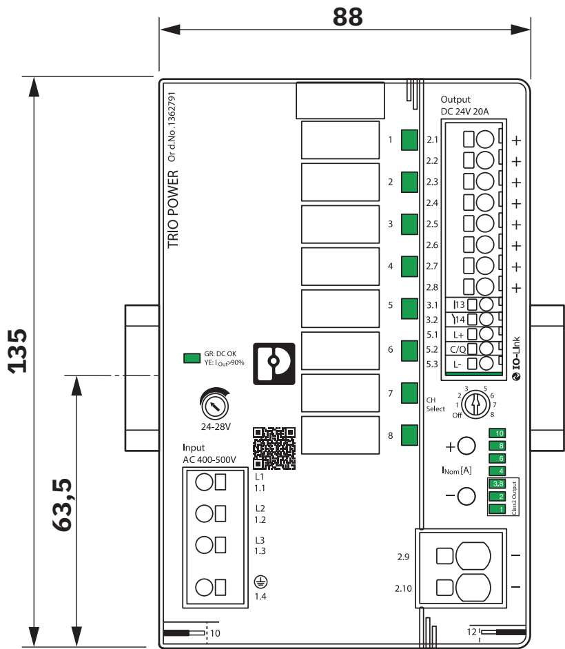
Disegno quotato
