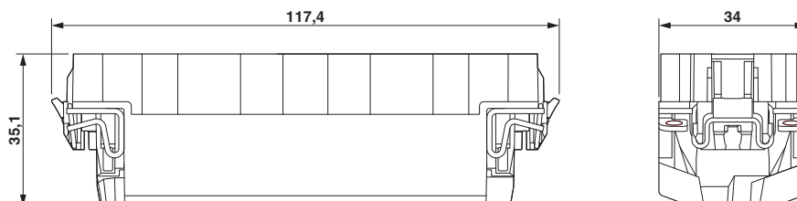
Disegno quotato
