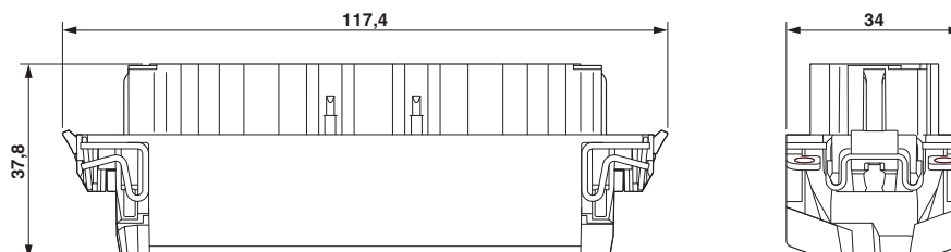
Disegno quotato
