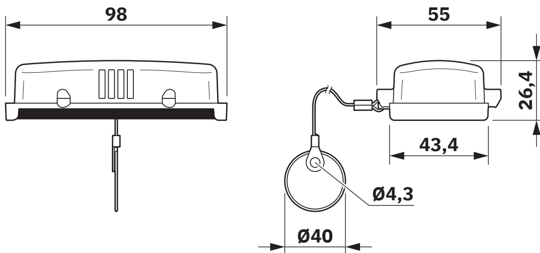
Disegno quotato
