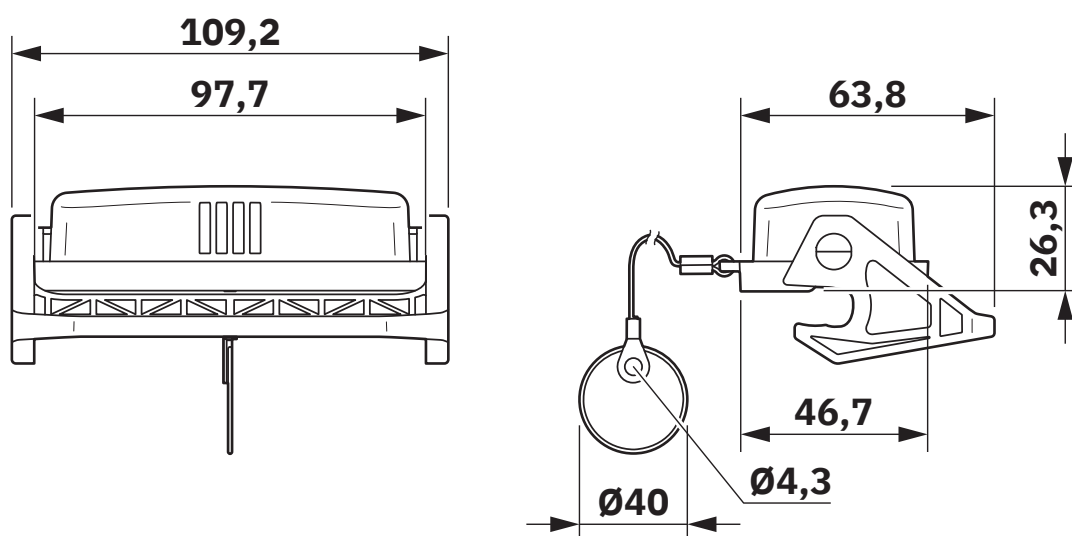
Disegno quotato
